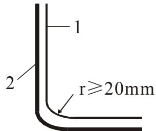
图 4.2.1 构件角处粘贴示意
