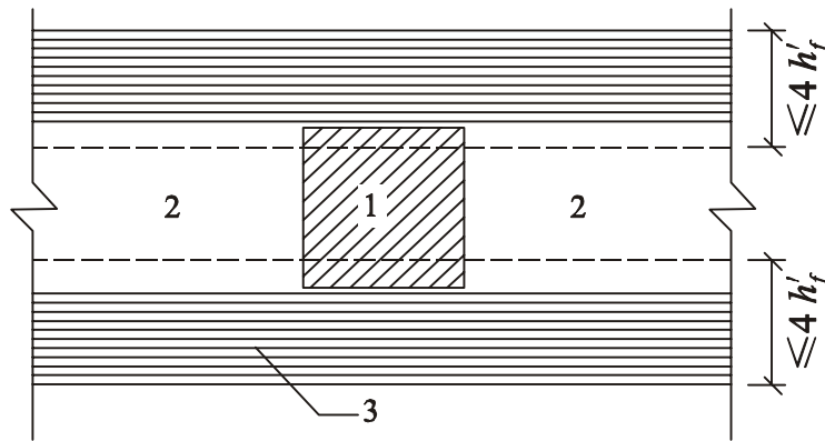
图 4.3.10 负弯矩区加固时梁侧有效粘贴范围平面图
