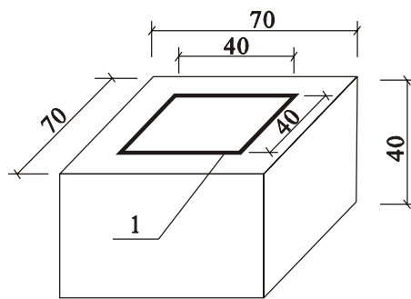
图 A.2.3 混凝土试块尺寸
